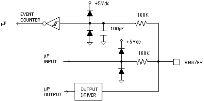
Figure 2.4 D1711, D1712 Events Counter Circuit.
